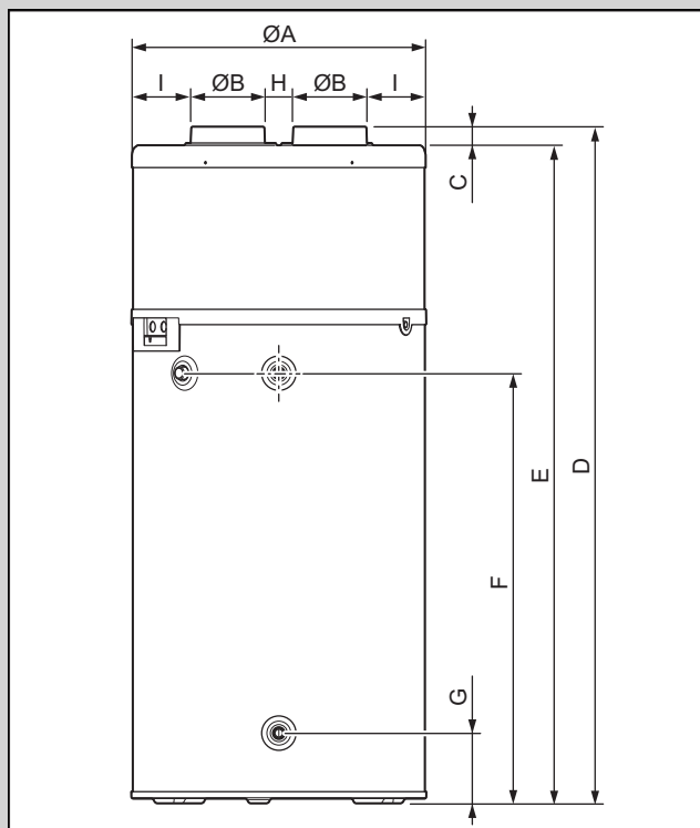
Dimensions de l'appareil et cotes de raccordement
