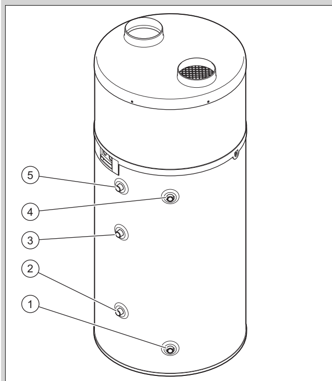
1 Raccord d'eau froide 2 Raccord sortie eau chauffage d'appoint
